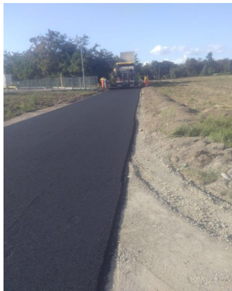
Przebudowa drogi gminnej Nr 130628W w miejscowości Kacprówek
