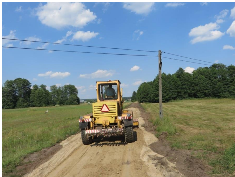
Remont drogi Nr 130630W w m. Dąbrowa
