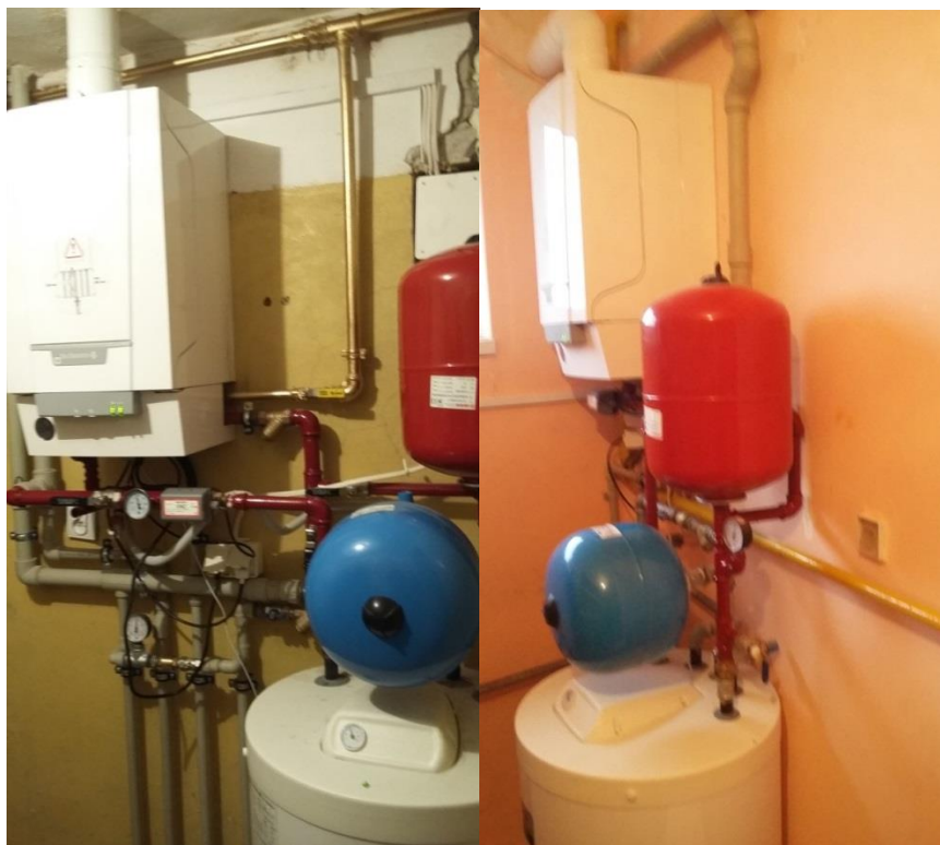
Systemy ogrzewania gazowego wykonane w świetlicach wiejskich w OSP Stary Pilczyn (z lewej) i OSP Wola Łaskarzewska (z prawej)
